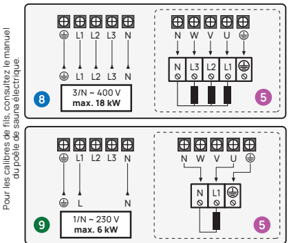
Figure 1. Connexions électriques de l'appareil.
