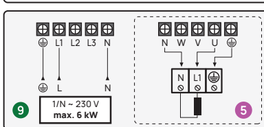
Joonis 1. Ühenduskeem.
